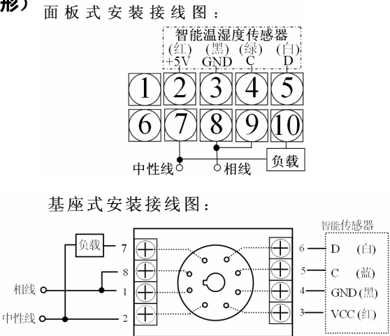
接线图
